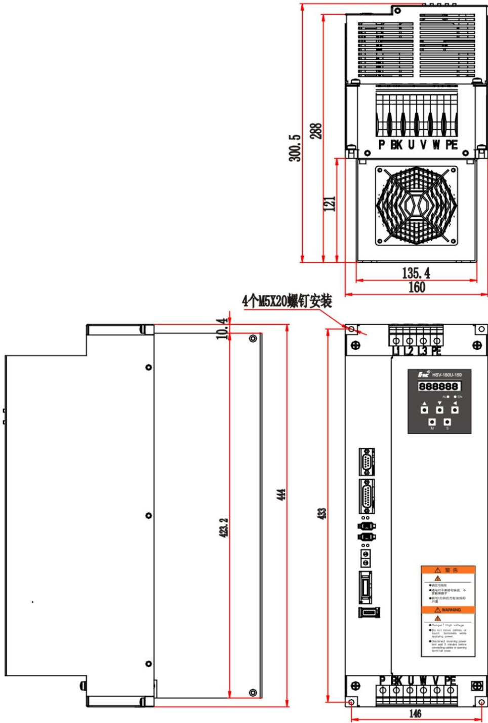
图 3.4 HSV-180UD-100, 150 伺服驱动单元外形尺寸 (未带辅助安装装置 单位: mm)
