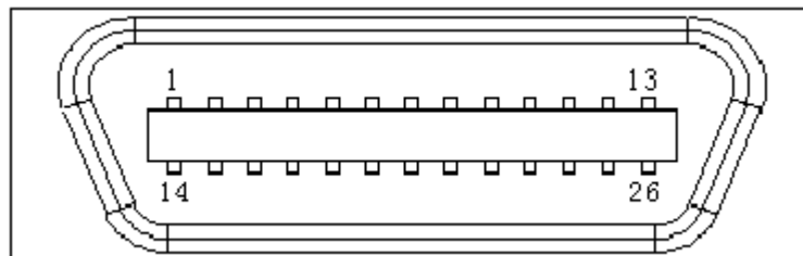
图 5.19 XS5 伺服电机编码器输入接口插头 (面对插头看)
