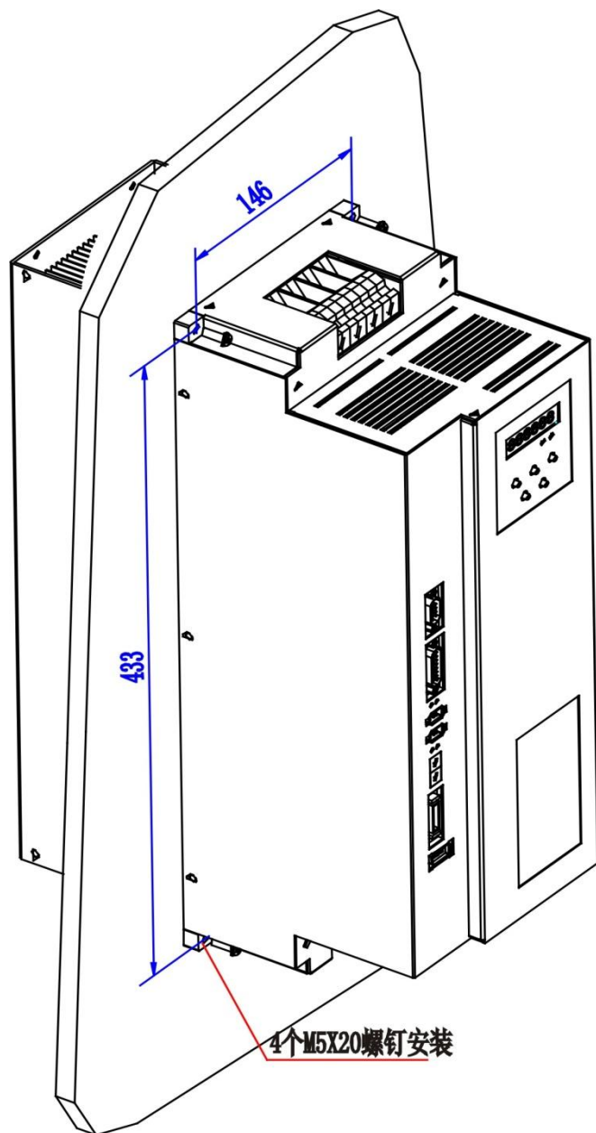
图 4.8 HSV-180UD-100, 150 驱动单元穿墙式安装示意图 (单位: mm)
