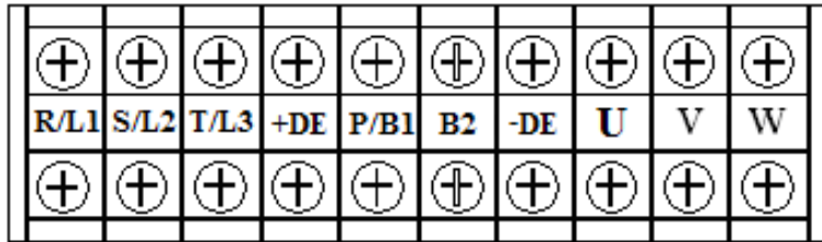
图 5.7 HSV-180U1D-200, 300 主回路端子
