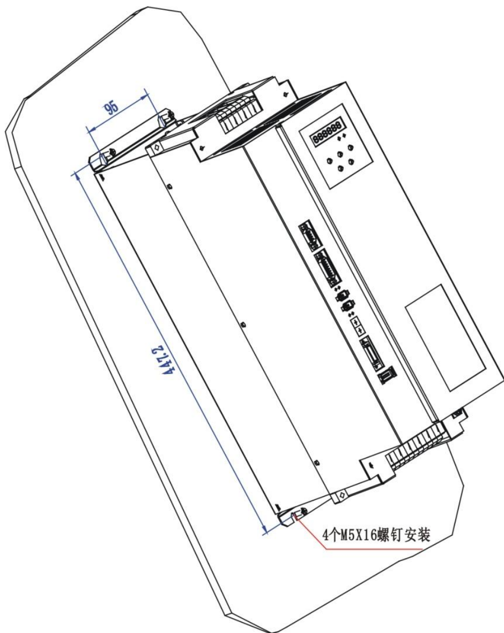
图 4.7 HSV-180UD-100, 150 驱动单元墙面安装示意图 (使用辅助安装装置 单位: mm)
