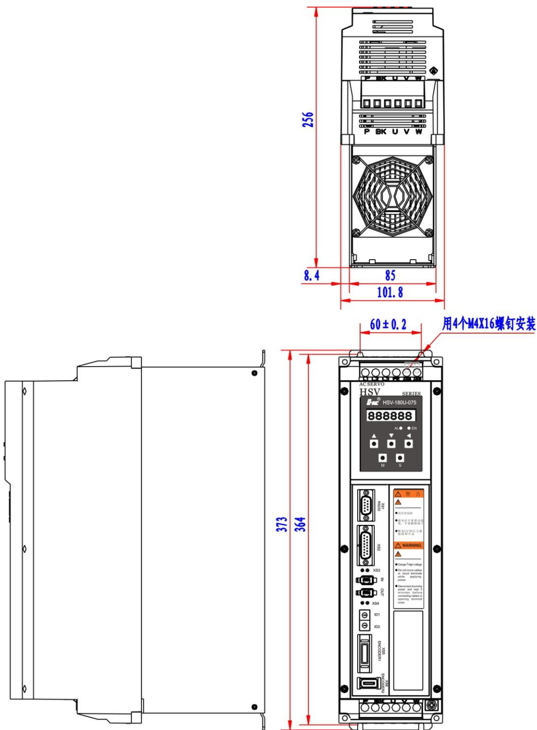
图 3.3 HSV-180UD-035, 050, 075 伺服驱动单元外形尺寸 (带辅助安装装置 单位: mm)
