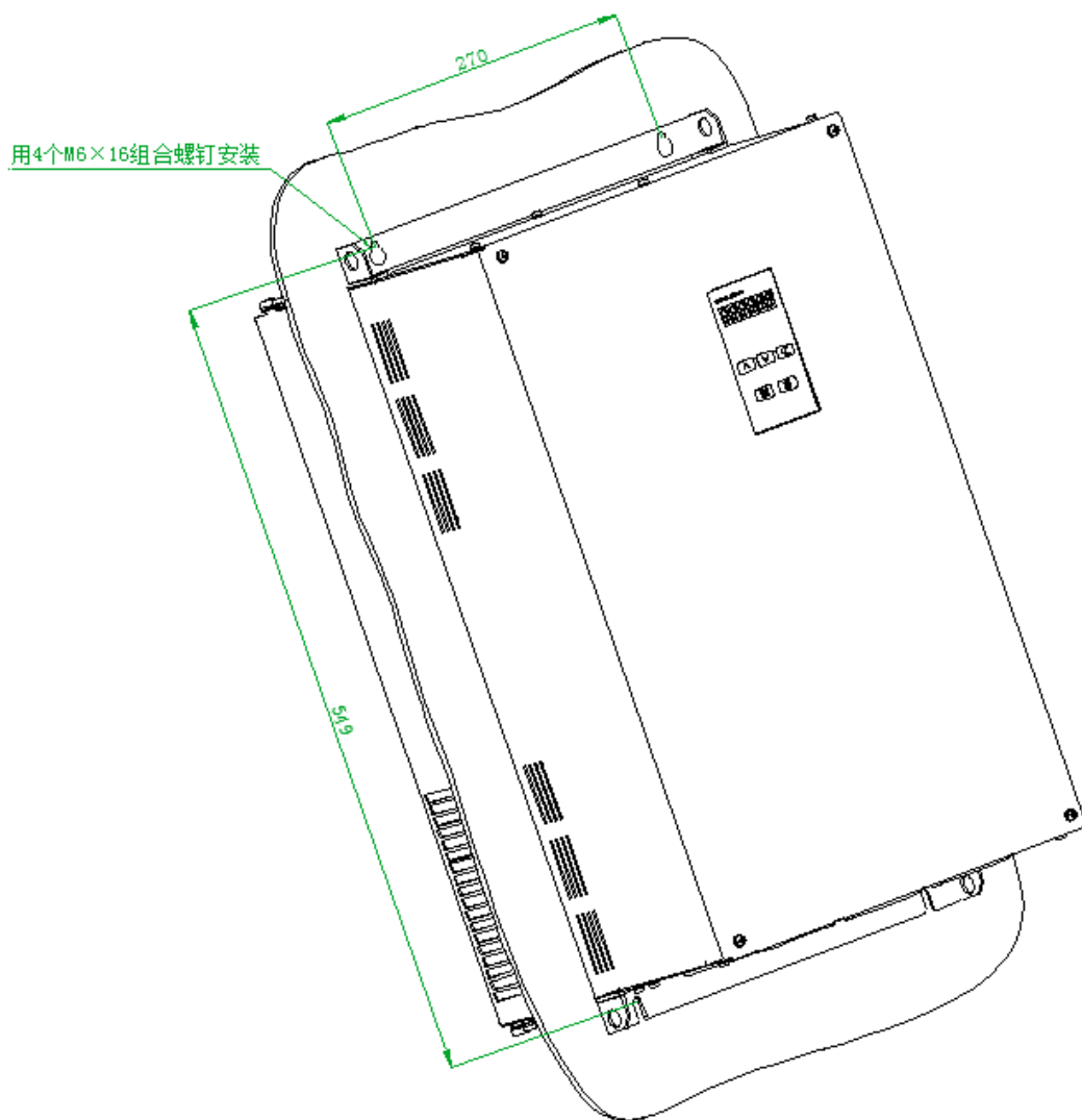
图 4. 23 HSV-180U1D-200, 300 驱动单元穿墙式安装示意图 (单位: mm)
