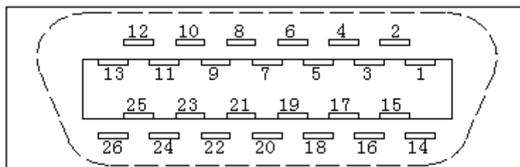
图 5.20 XS5 伺服电机编码器输入接口插头的焊接脚 (面对插头的焊接脚看)
