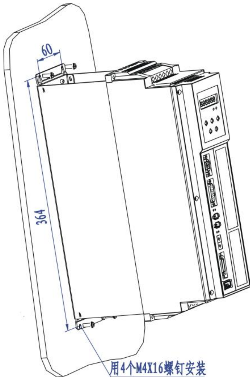
图 4.2 HSV-180UD-035, 050, 075 驱动单元墙面安装示意图 (使用辅助安装装置 单位: mm)
