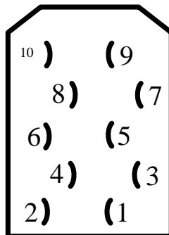
图 5.30 XS6 ENCODER2 第二位置编码器输入接口插头的焊接脚(面对插头的焊接脚看)
