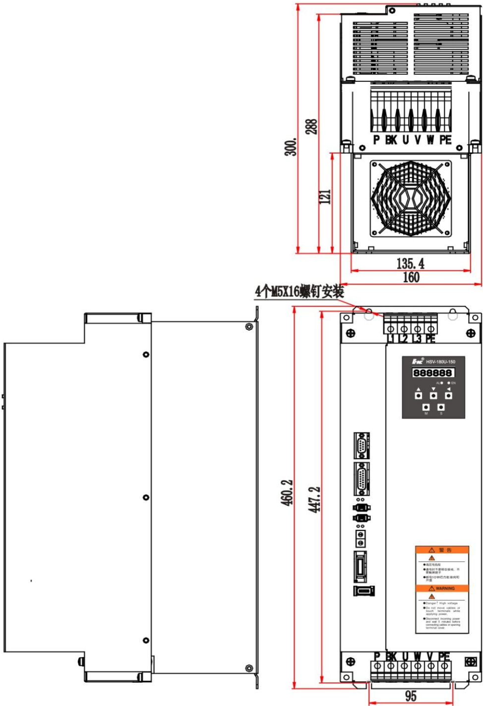
图 3.5 HSV-180UD-100, 150 伺服驱动单元外形尺寸（带辅助安装装置 单位：mm）
