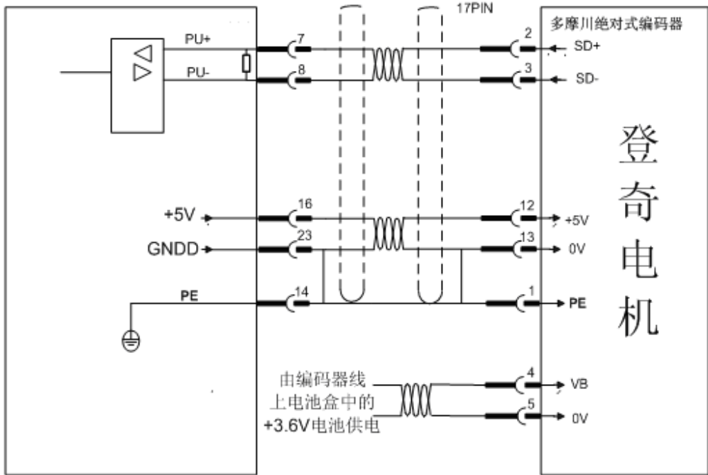
图 5.26 伺服驱动单元与安装 TAMAGAWA 协议编码器登奇电机接线图
