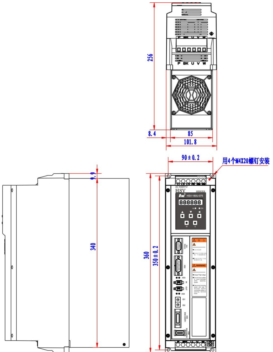
图 3.2 HSV-180UD-035, 050, 075 伺服驱动单元外形尺寸（未带辅助安装装置 单位：mm）
