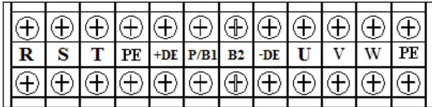
图 5.6 HSV-180U1D-100, 150 主回路端子
