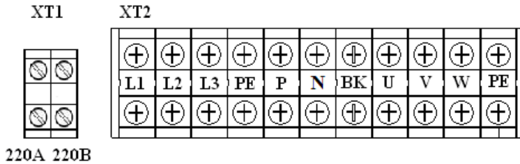
图 5.5 HSV-180UD-200, 300, 450 主回路端子
