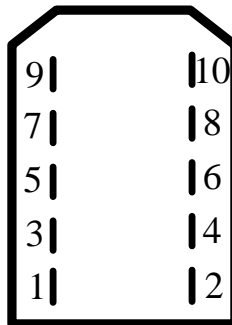
图 5.29 XS6 ENCODER2 第二位置编码器输入接口插头(面对插头看)
