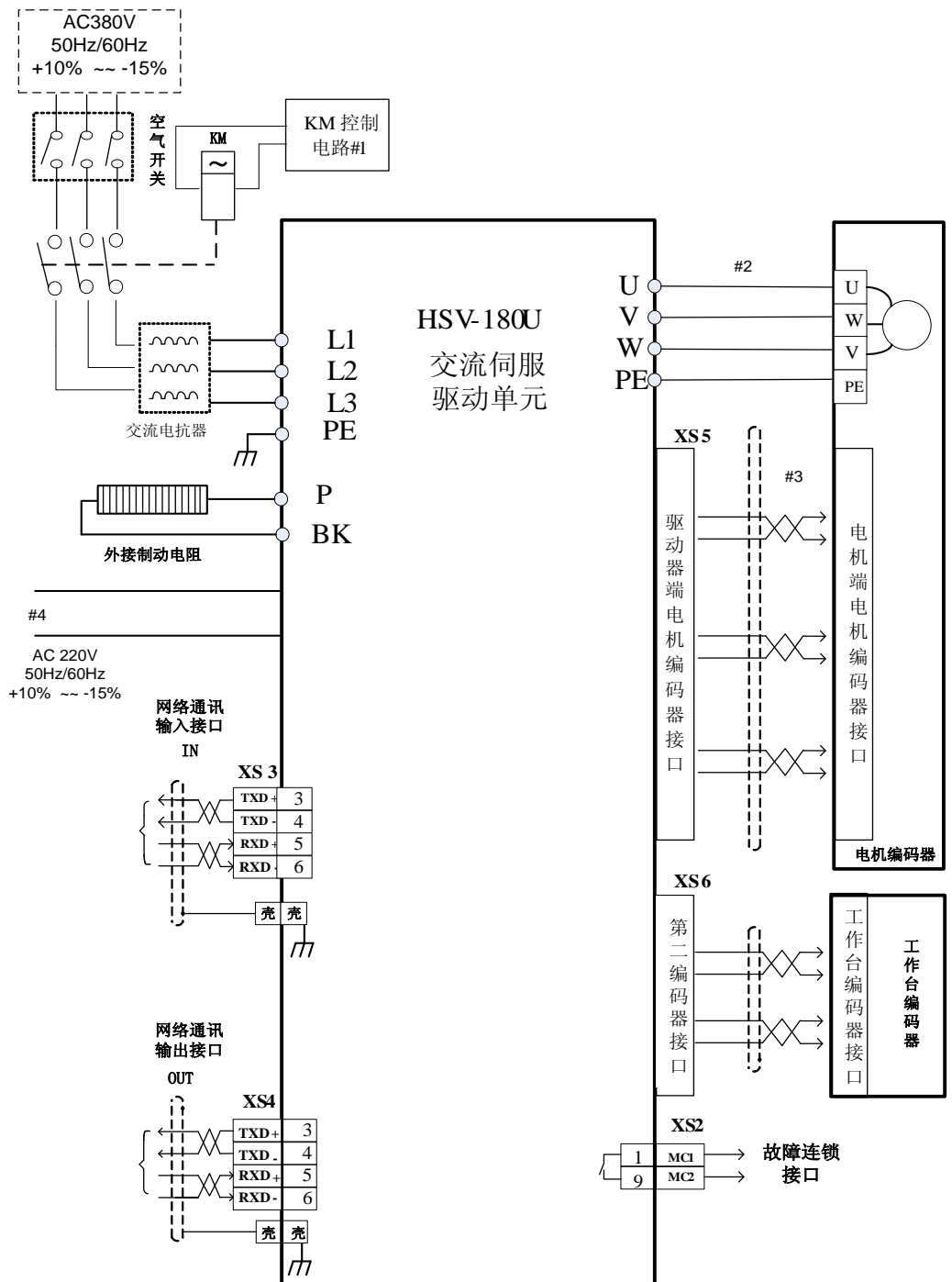
图 5.1 伺服驱动单元周边器件连接图
