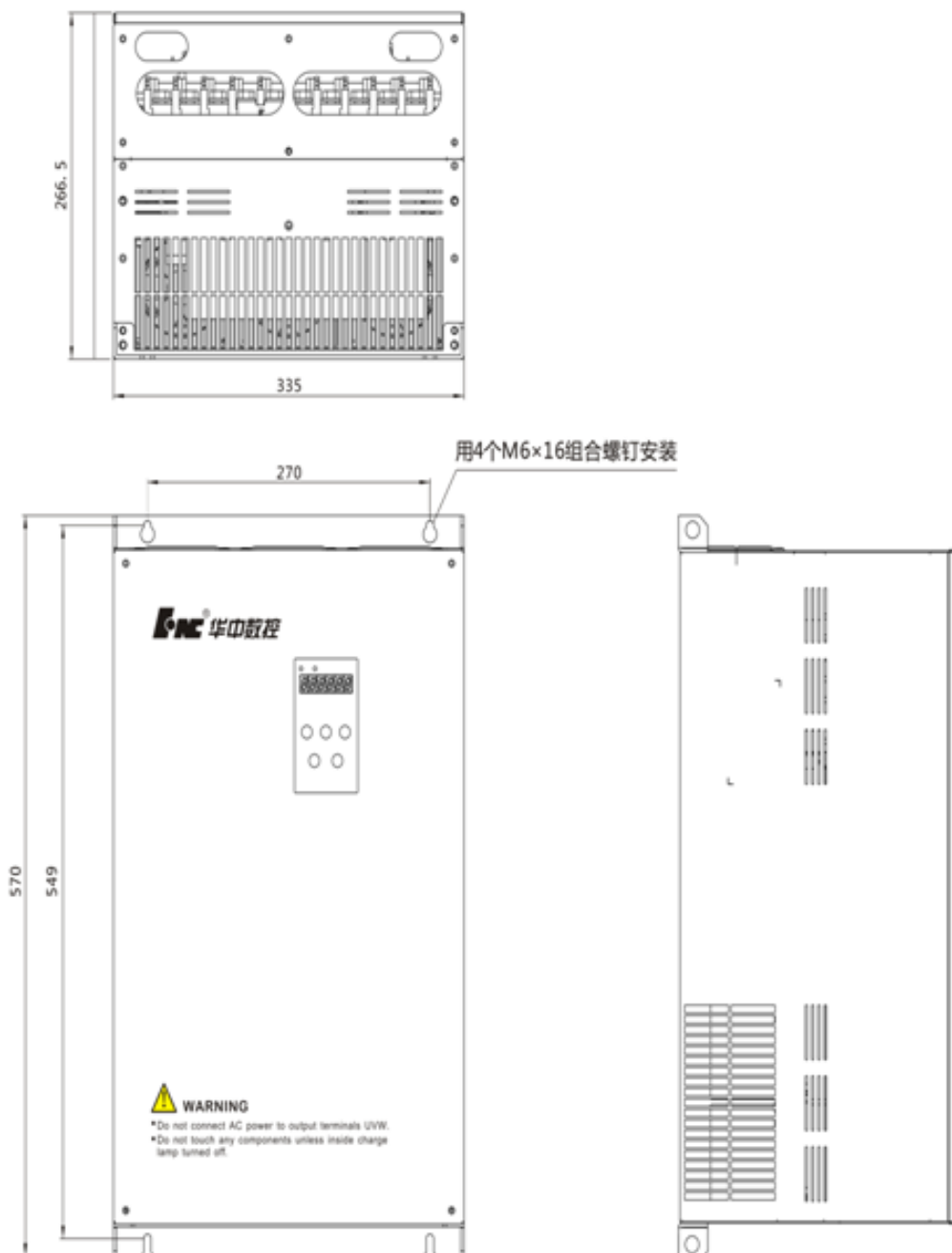
图 3.9 HSV-180U1D-200, 300 伺服驱动单元外形尺寸（带辅助安装装置 单位：mm）
