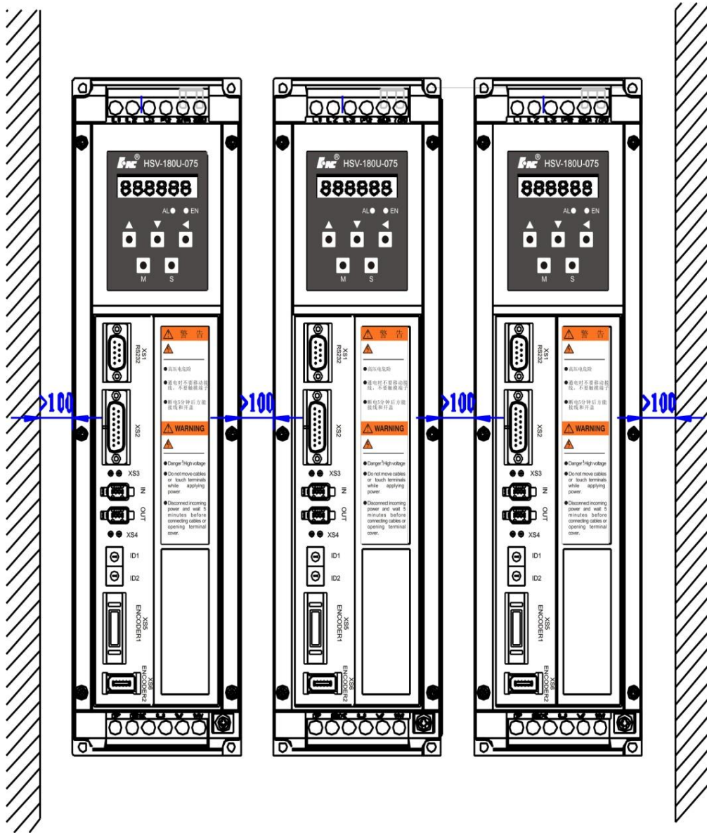
图 4.6 HSV-180UD-035, 050, 075 驱动单元多台安装间隔 (单位: mm)
