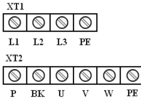
图 5.4 HSV-180UD-100,150 主回路端子
