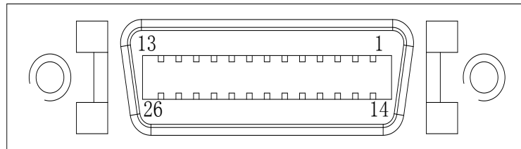
图 5.18 XS5 伺服电机编码器输入接口插座
