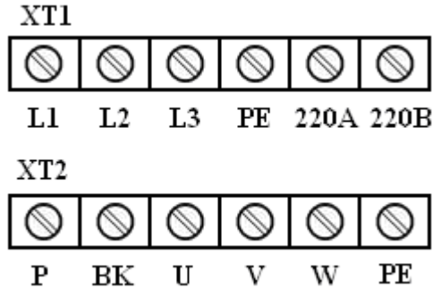
图 5.3 HSV-180UD-035,050,075 主回路端子
