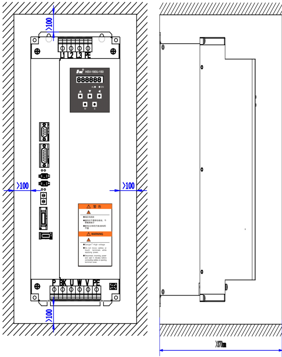
图 4.9 HSV-180UD-100, 150 驱动单元单台安装间隔 (墙面安装 单位: mm)
