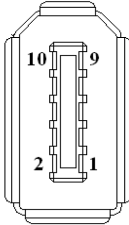
图 5.28 XS6 ENCODER2 第二位置编码器输入接口插座
