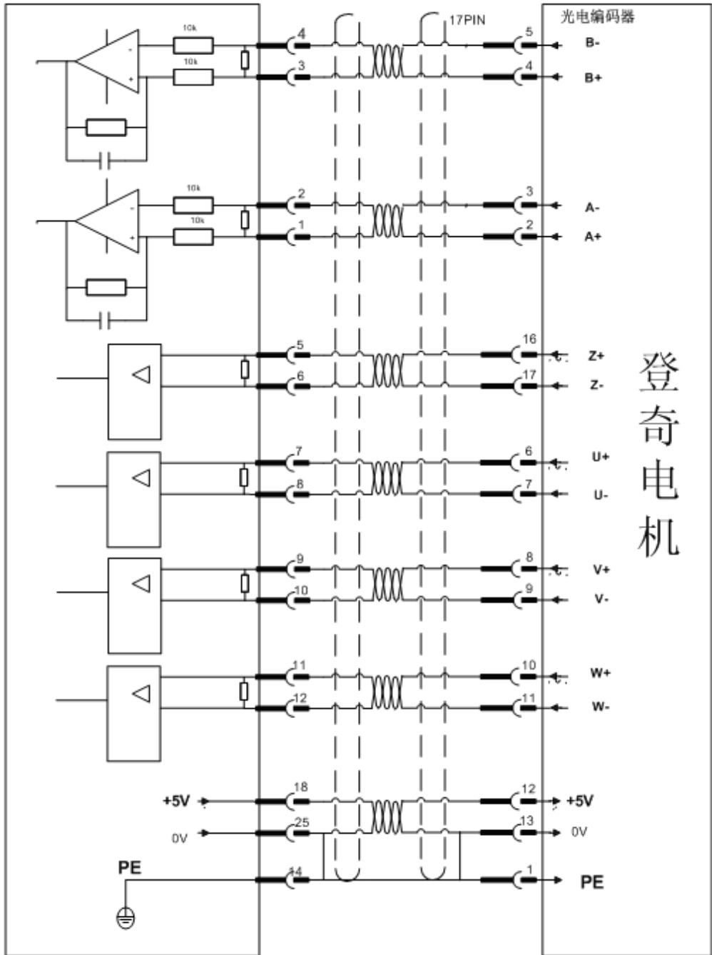
图 5.21 伺服驱动单元与安装复合增量式光电编码器登奇电机接线图
