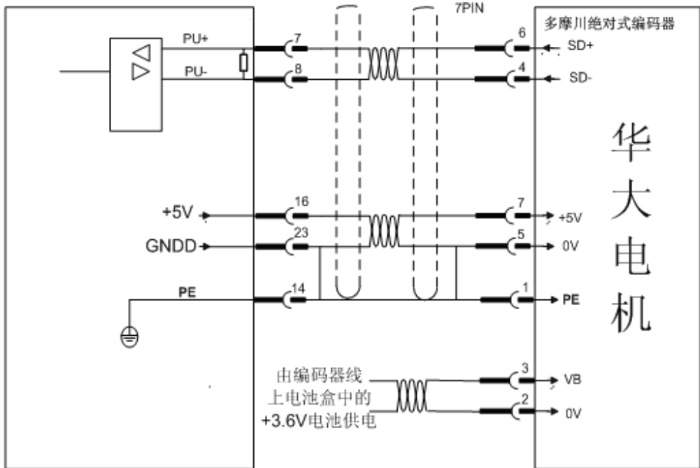
图 5.27 伺服驱动单元与安装 TAMAGAWA 协议编码器华大电机接线图
